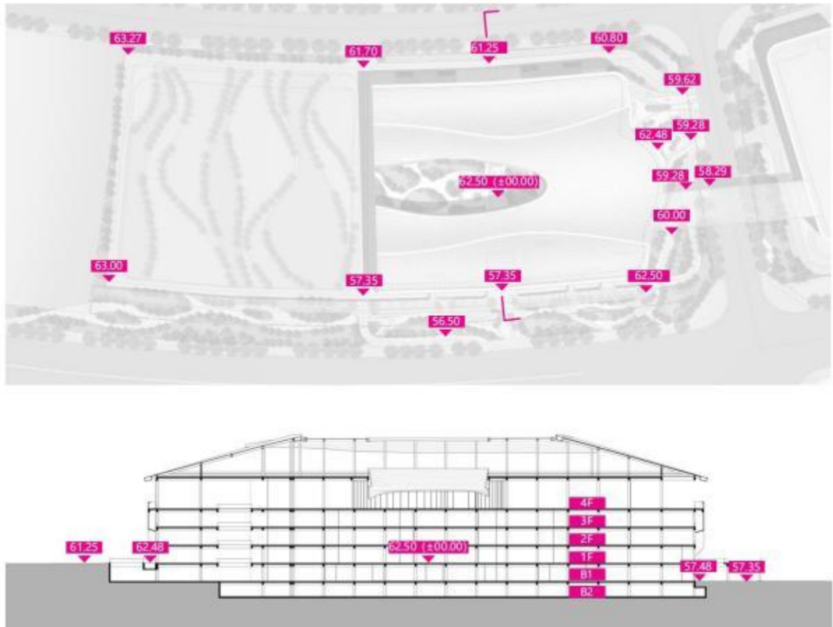
1-3 项目竖向设计分析图
